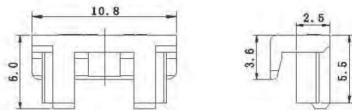
B600003-5-02A MG610228 止档片
