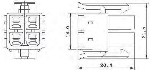
B600003-5-02B MG610228 锁定片
