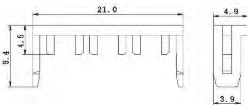
B600003-5-03B MG610226 锁定片
