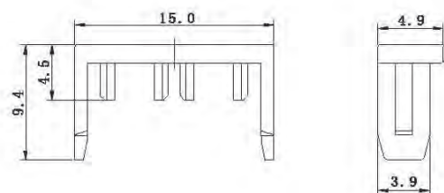
B600003-5-02B MG610228 锁定片
